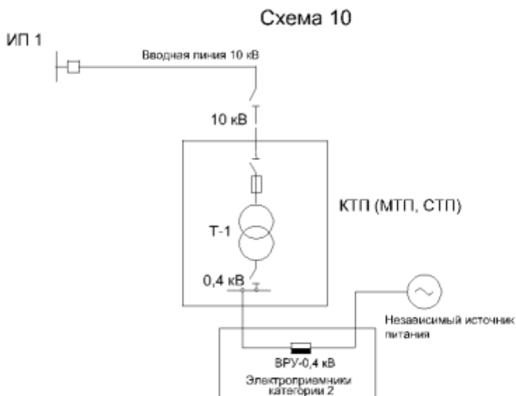
Рисунок 10 – Схема присоединения ТП 10/0,4 кВ, питающей потребителей категории 2
