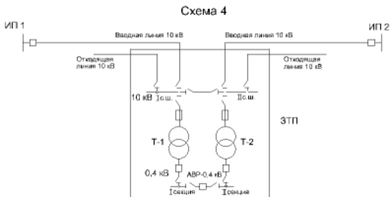
Рисунок 4 – Схема присоединения ТП 10/0,4 кВ, питающей потребителей категории 1
