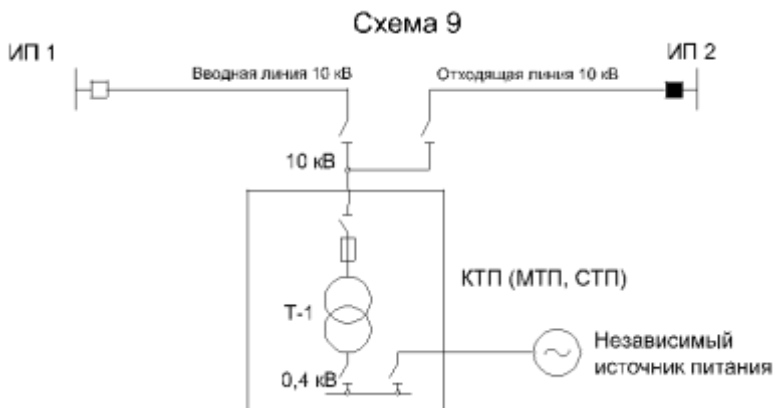
Рисунок 9 – Схема присоединения ТП 10/0,4 кВ, питающей потребителей категории 2
