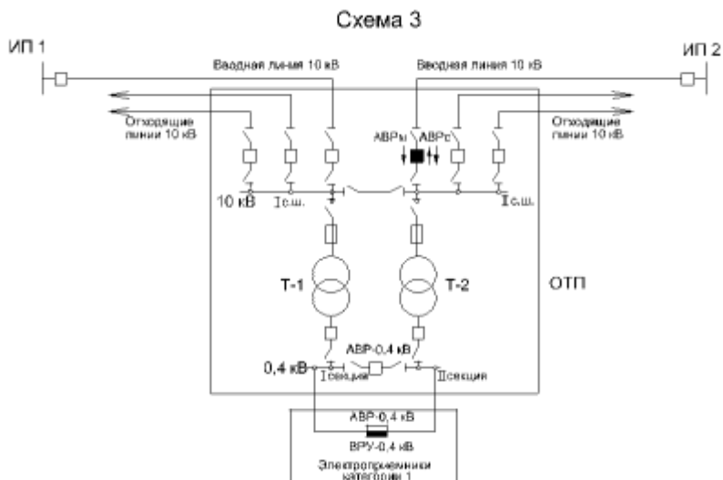
Рисунок 3 – Схема присоединения ТП 10/0,4 кВ, питающей потребителей категории 1
