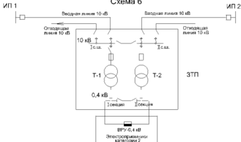
Рисунок 6 – Схема присоединения ТП 10/0,4 кВ, питающей потребителей категории 2
