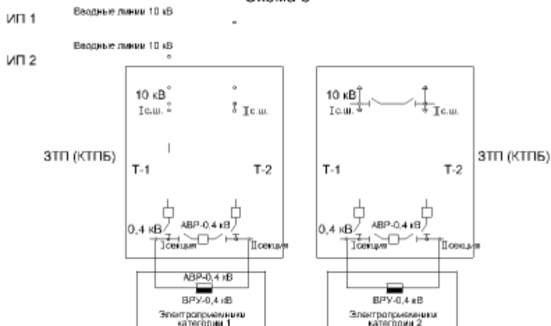
Рисунок 5 – Схема присоединения ТП 10/0,4 кВ, питающей потребителей категорий 1 и 2
